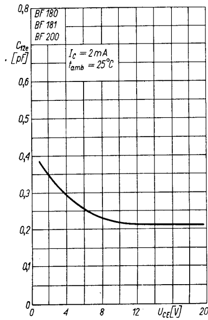
Zależność pojemności sprzężenia zwrotnego od napięcia C_{12es} = f(U_{CE})
