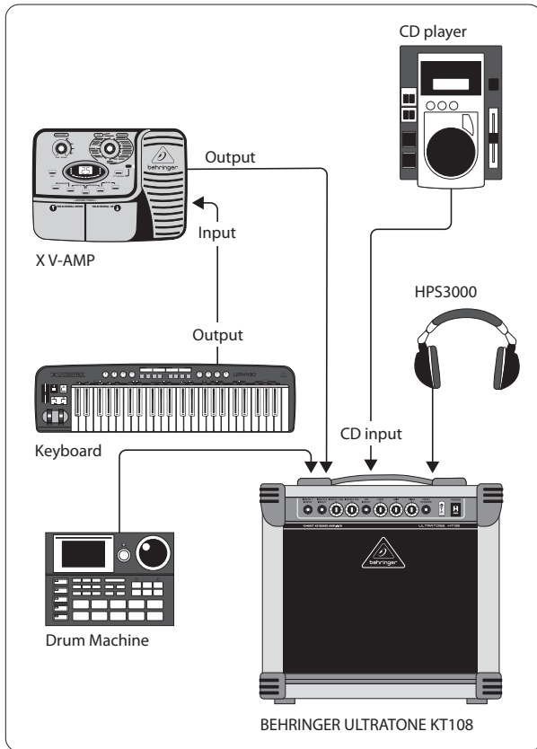
Fig. 2.1: Ejemplo de conexión para el ULTRATONE KT108
