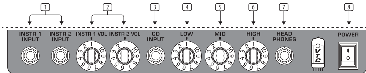
Fig. 3.1: Elementos de control en el panel frontal
